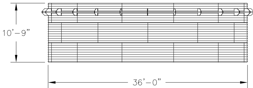
ELEVATION
