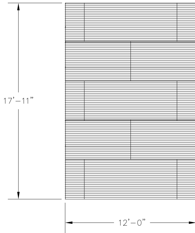
ELEVATION
