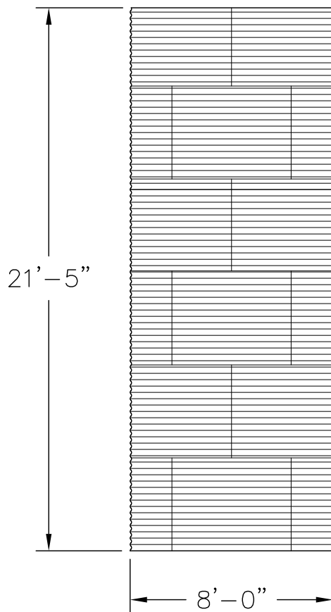
ELEVATION
