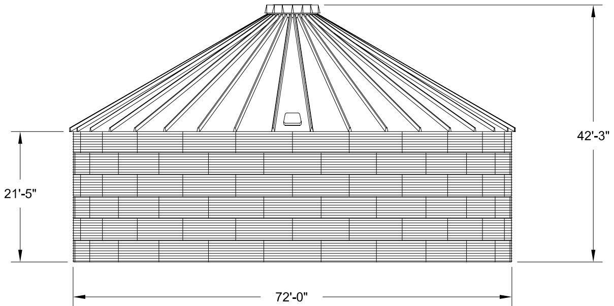
ELEVATION
