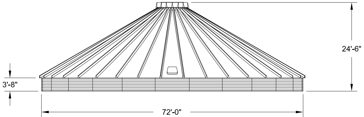
ELEVATION
