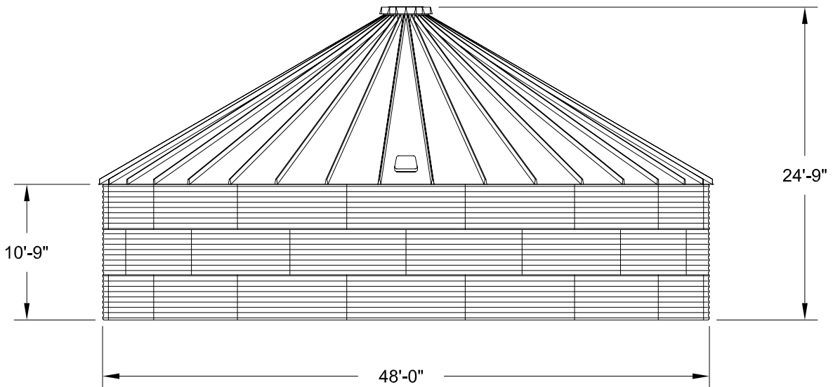
ELEVATION
