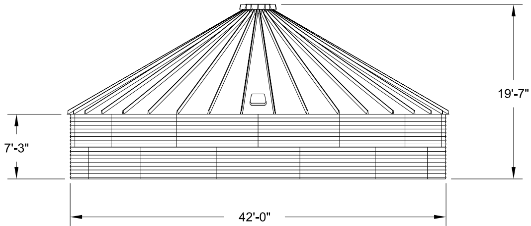
ELEVATION
