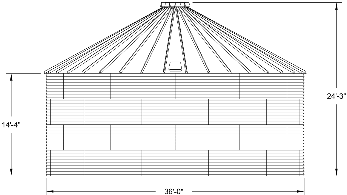
ELEVATION
