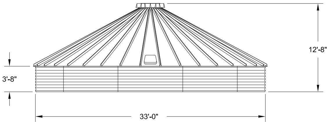
ELEVATION
