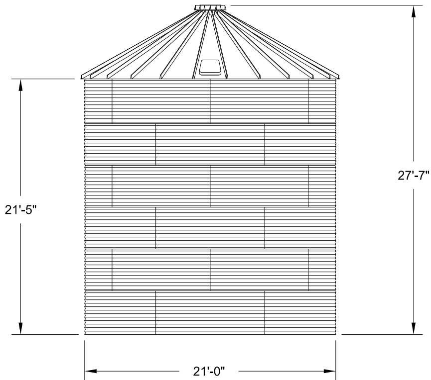
ELEVATION
