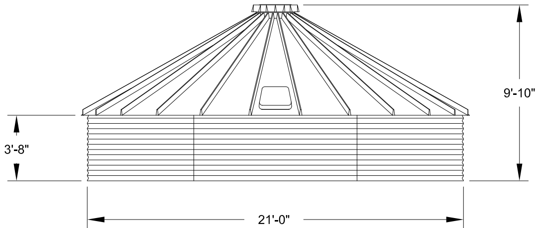
ELEVATION
