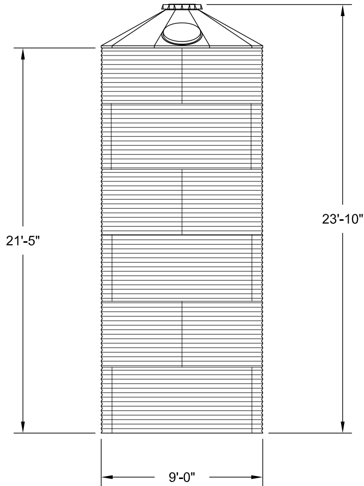
ELEVATION
