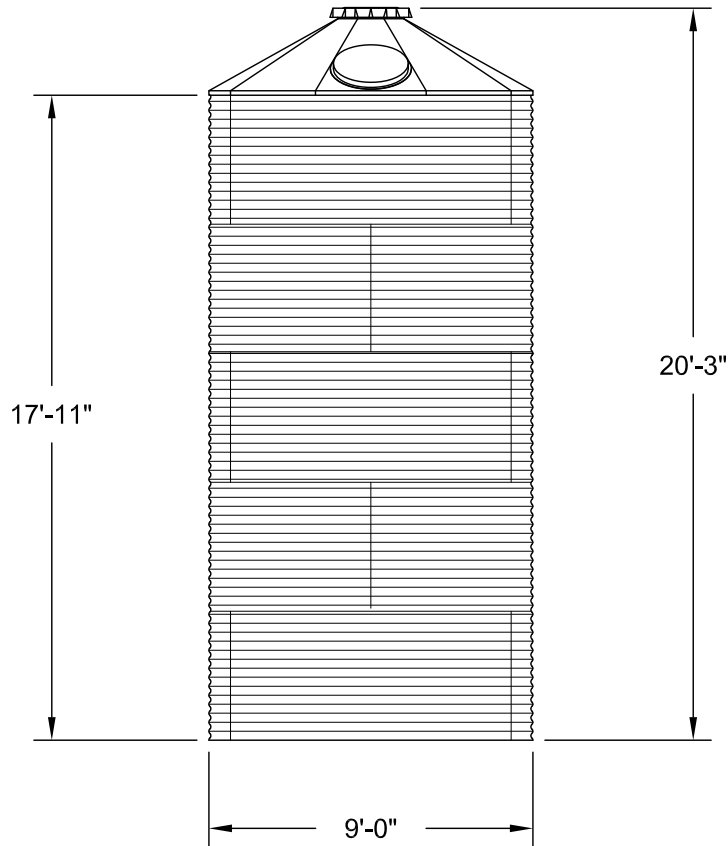
ELEVATION
