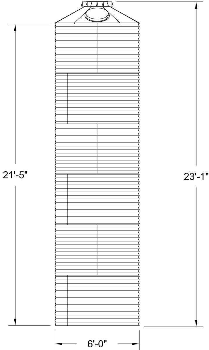
ELEVATION
