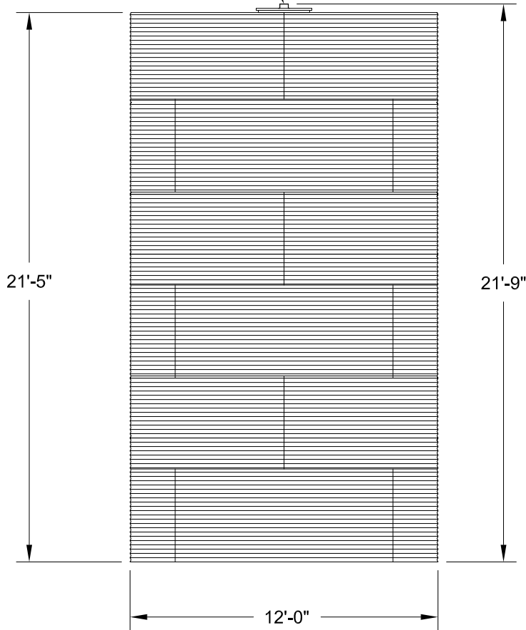
ELEVATION
