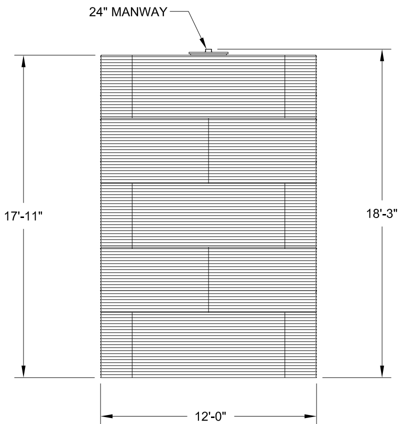
ELEVATION
