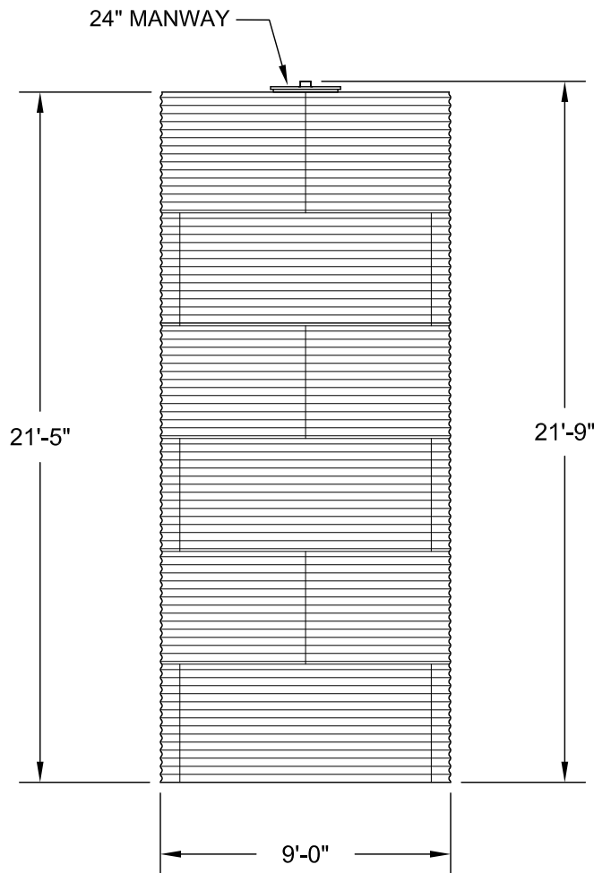
ELEVATION
