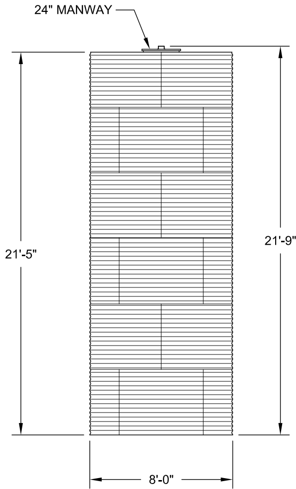
ELEVATION
