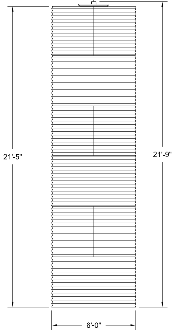
ELEVATION
