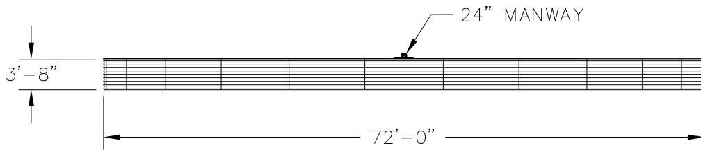
ELEVATION
