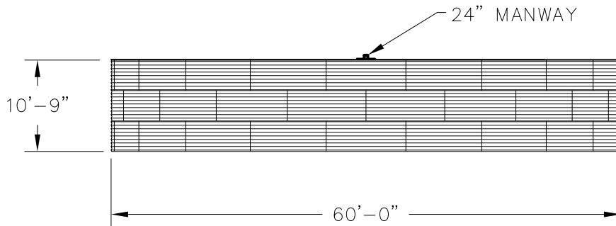
ELEVATION
