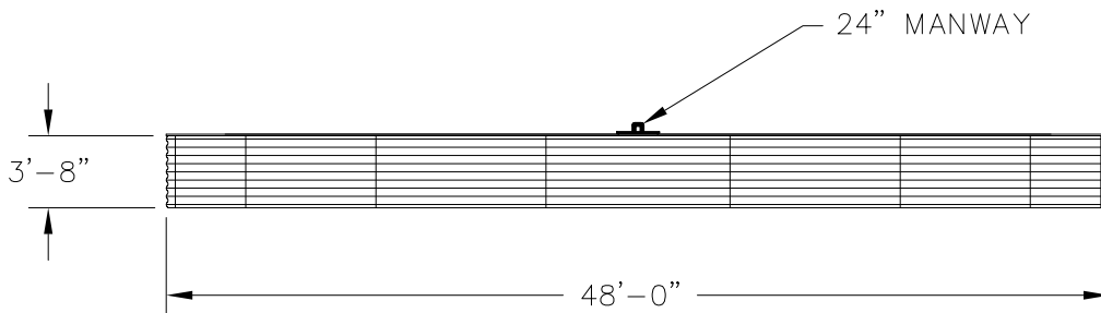
ELEVATION
