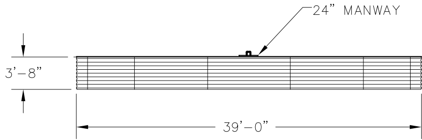
ELEVATION
