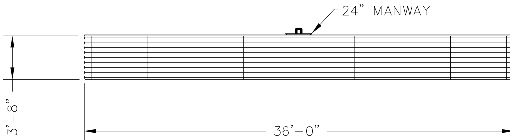
ELEVATION
