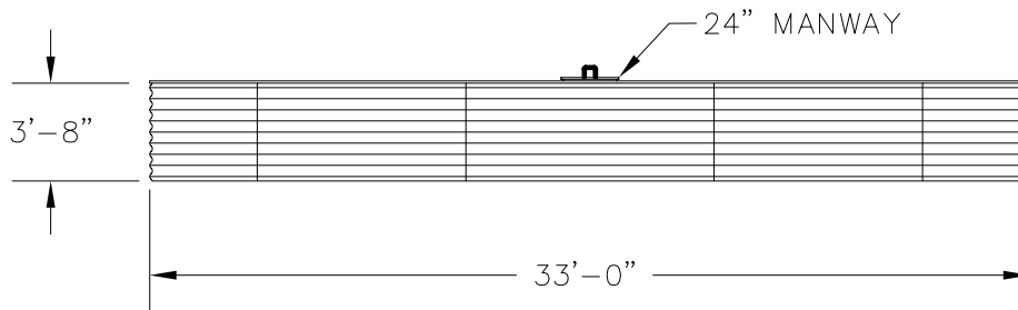
ELEVATION
