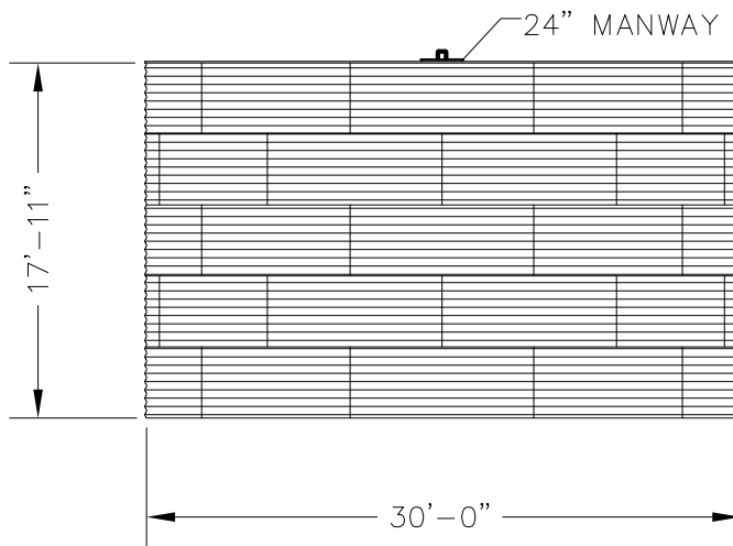
ELEVATION
