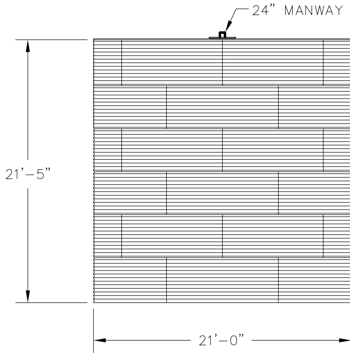
ELEVATION
