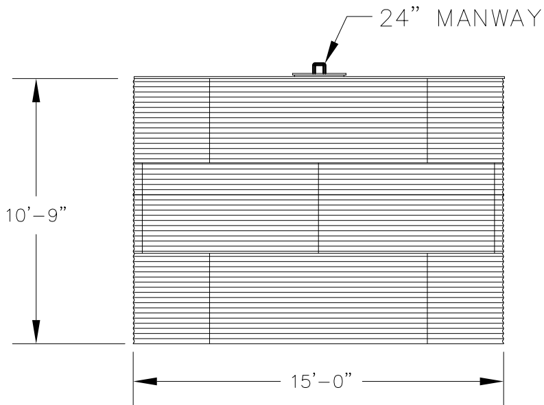
ELEVATION
