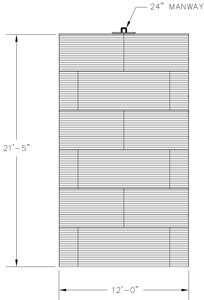
ELEVATION
